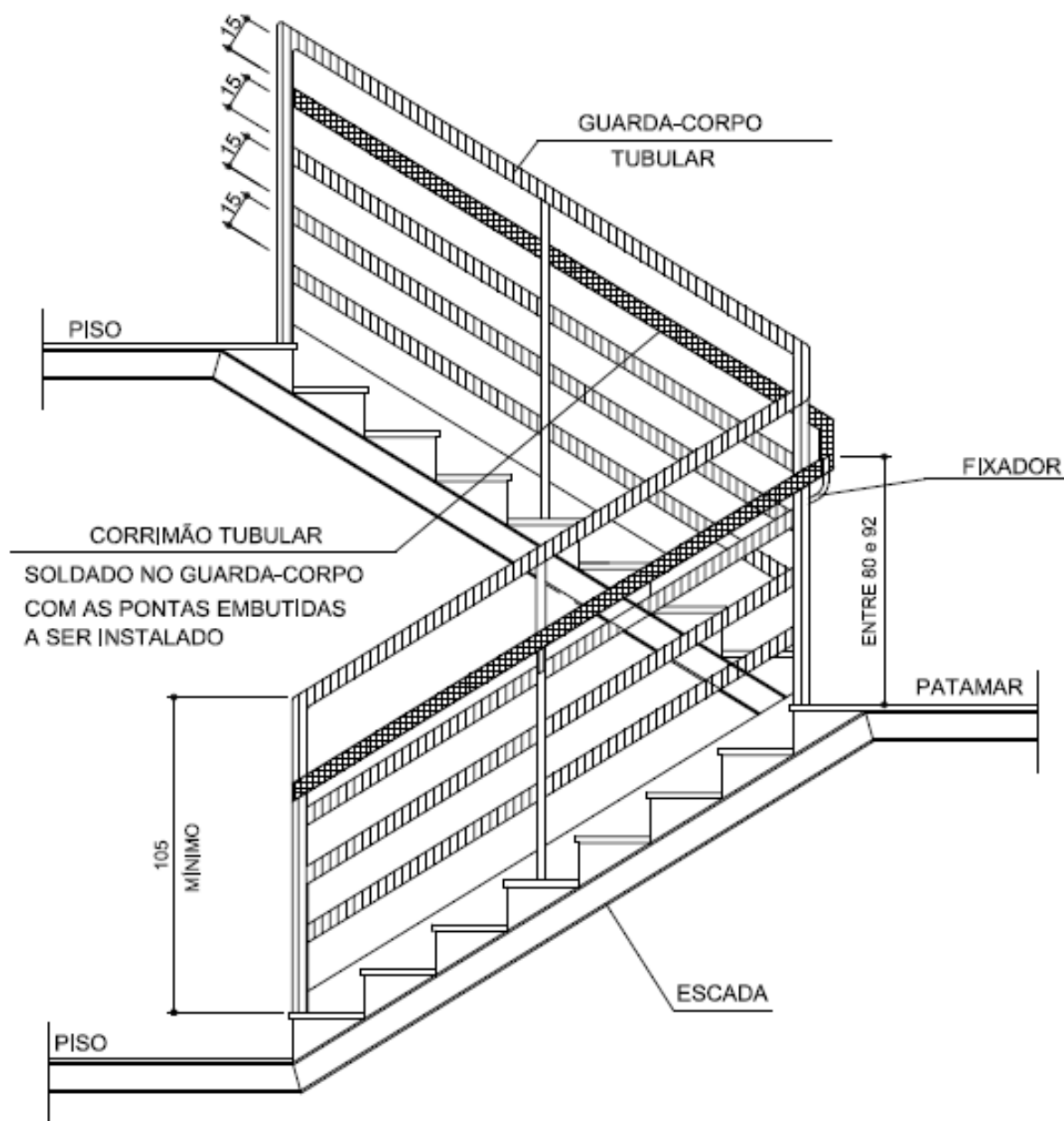
DETALHE GUARDA-CORPO ESCADA SEM ESCALA
